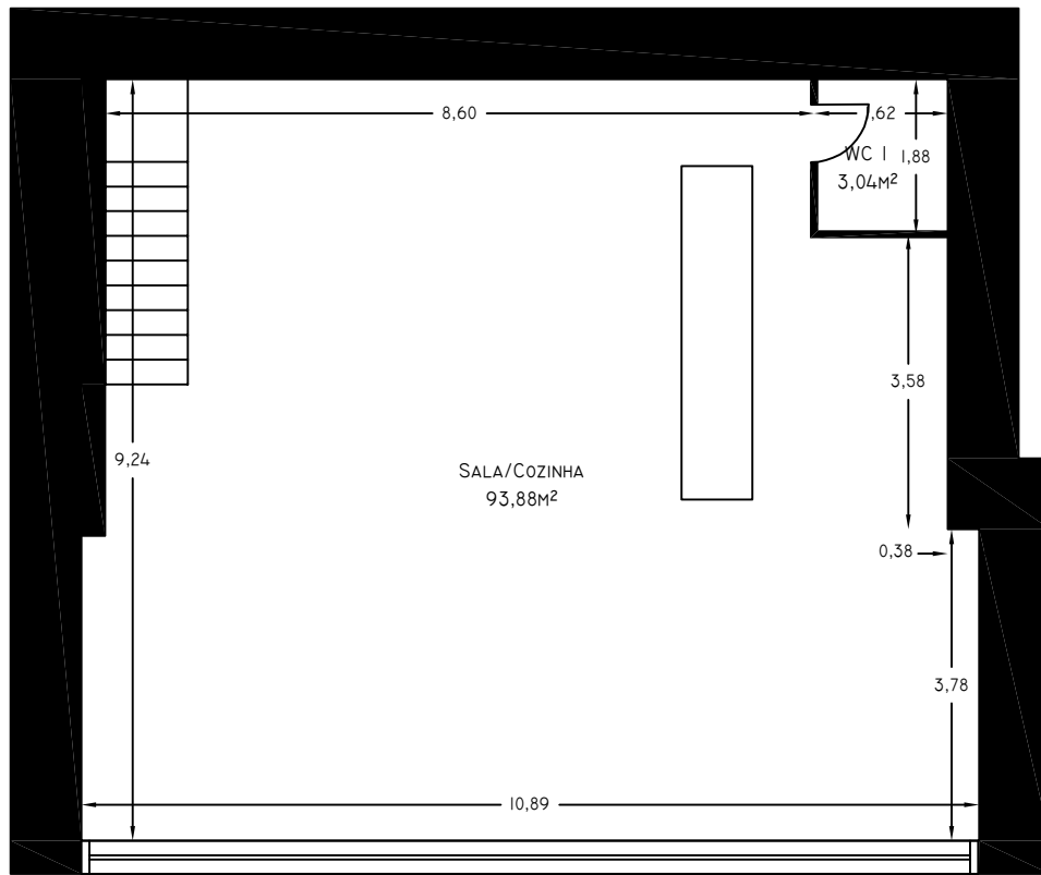
Planta Piso Rc
