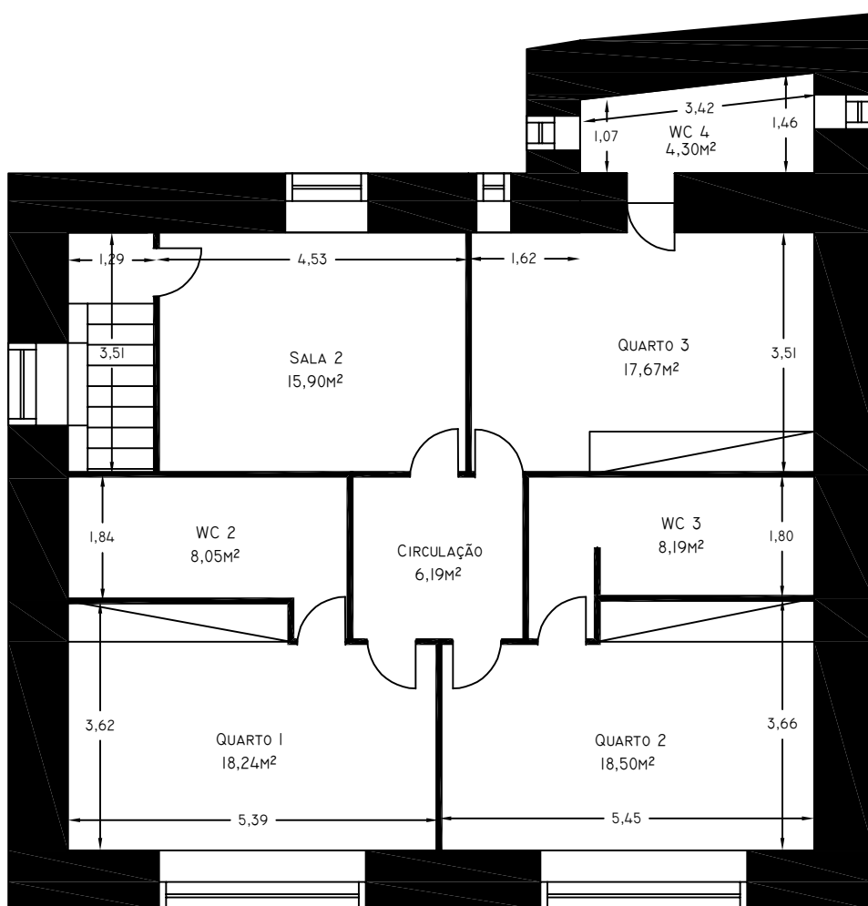
Planta Piso I
