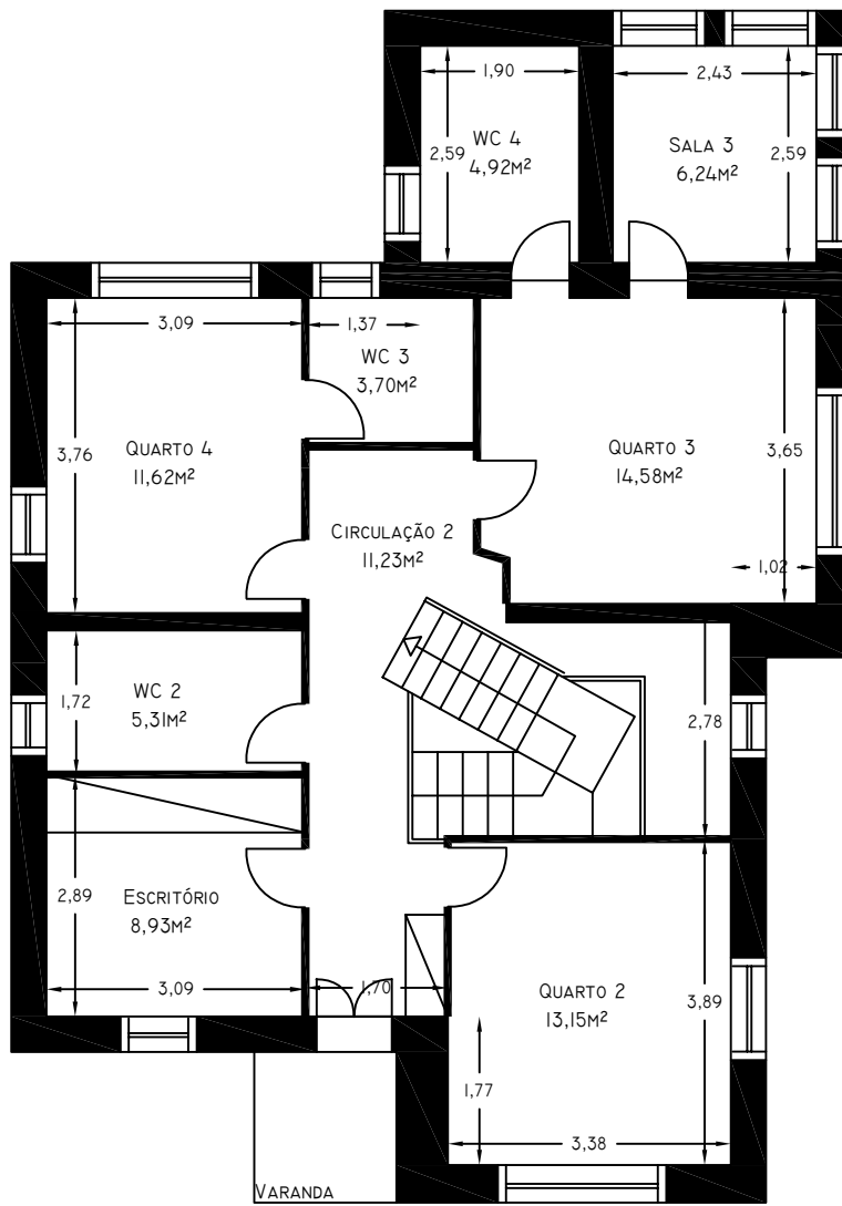
Planta Piso I
