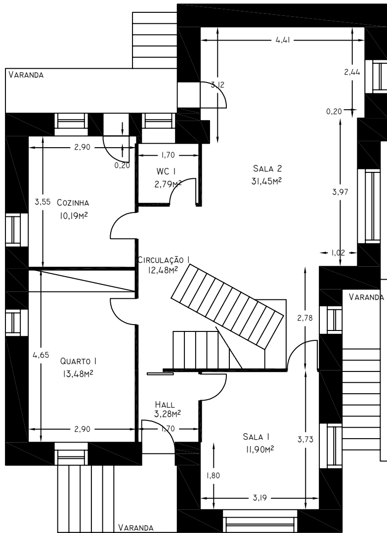
Planta Piso RC
