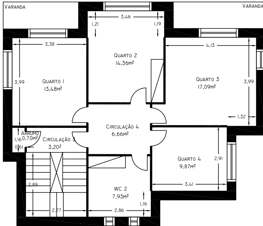
Planta Piso 1º Andar
