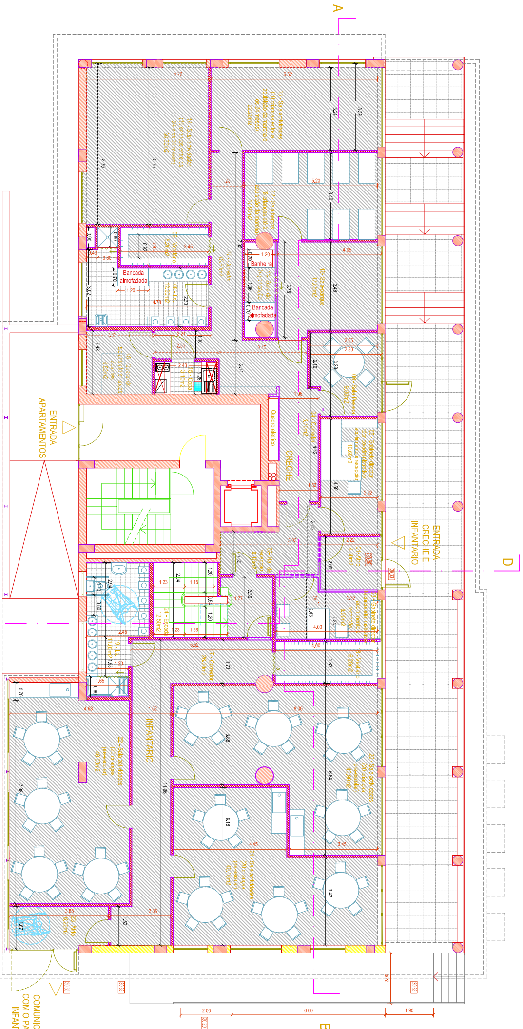
Planta do piso 1
