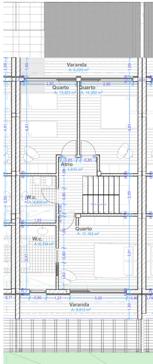
PLANTA DO PISO 1
