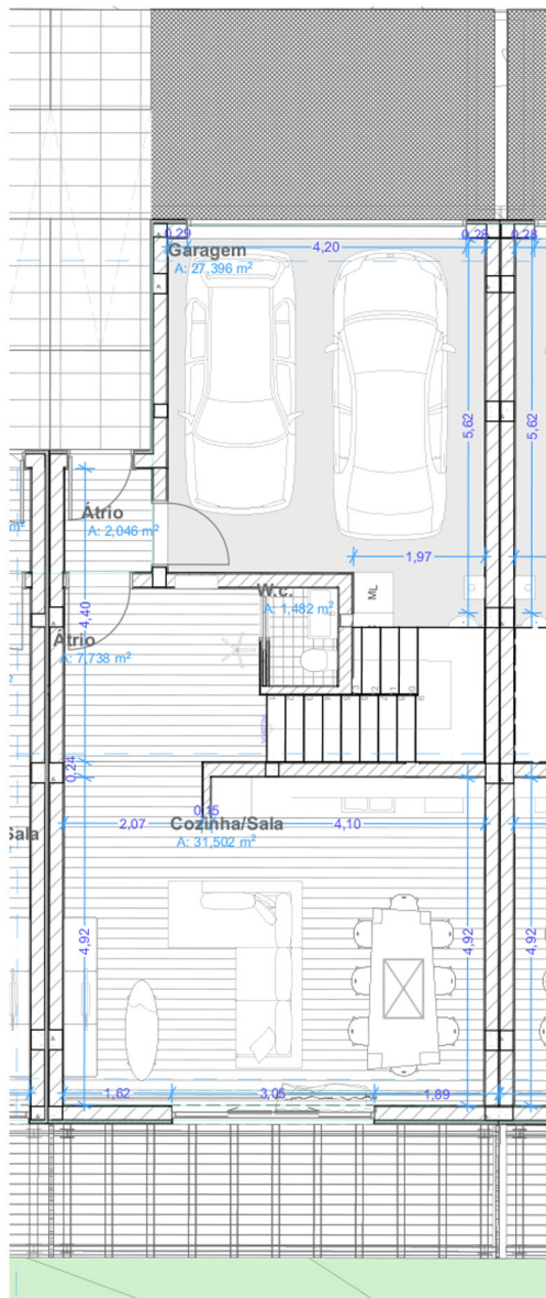
PLANTA DO PISO 0
