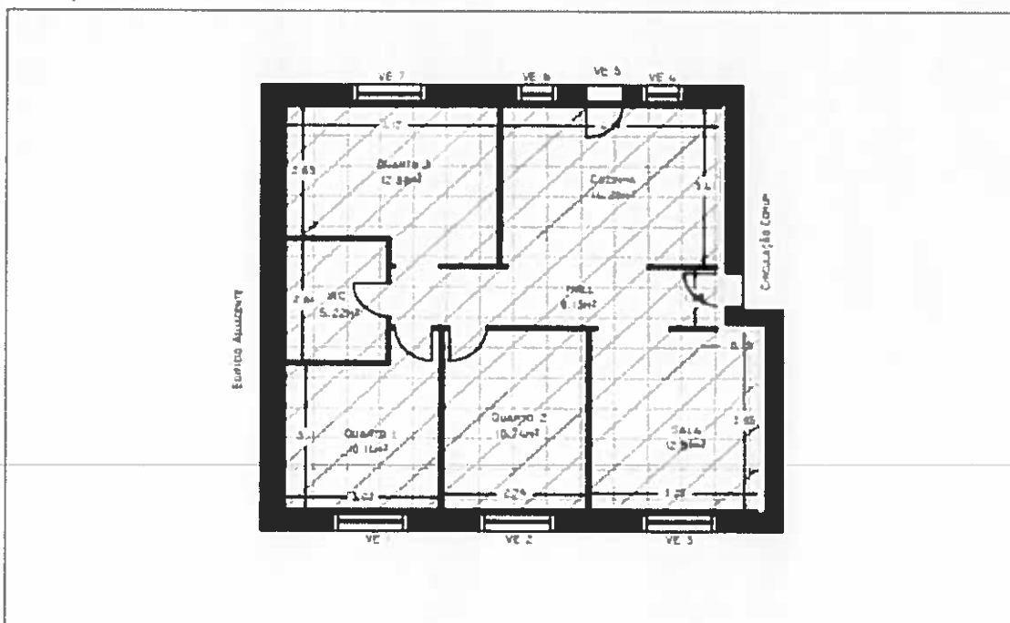
PLANTA Escala = 1:100
