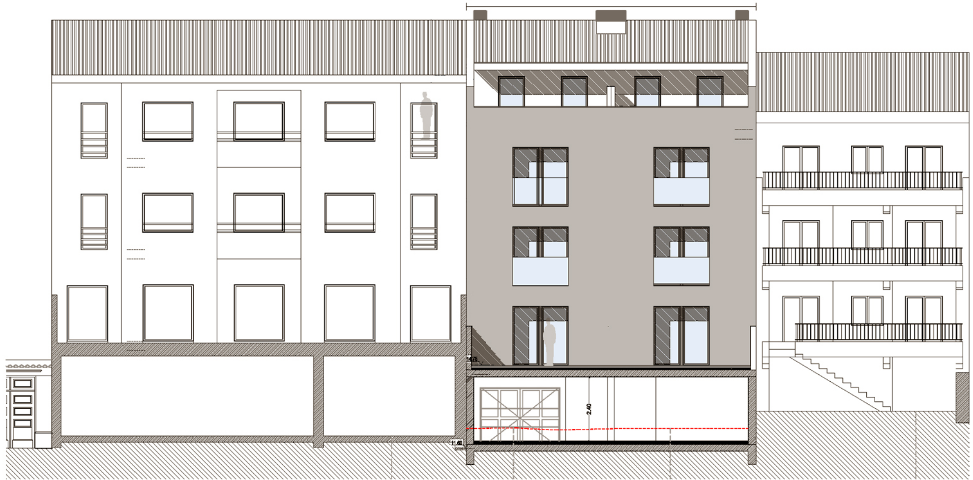
Alçado tardoz
