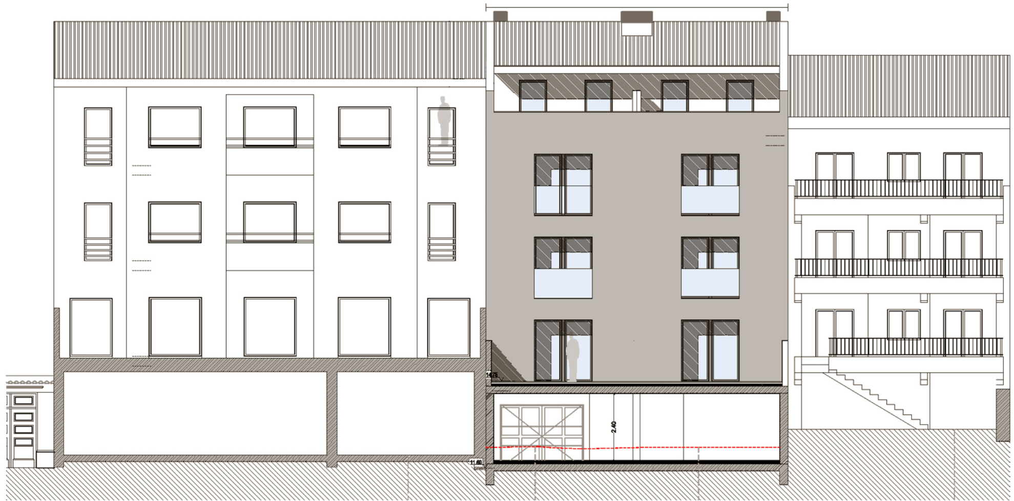
Alçado tardoz
