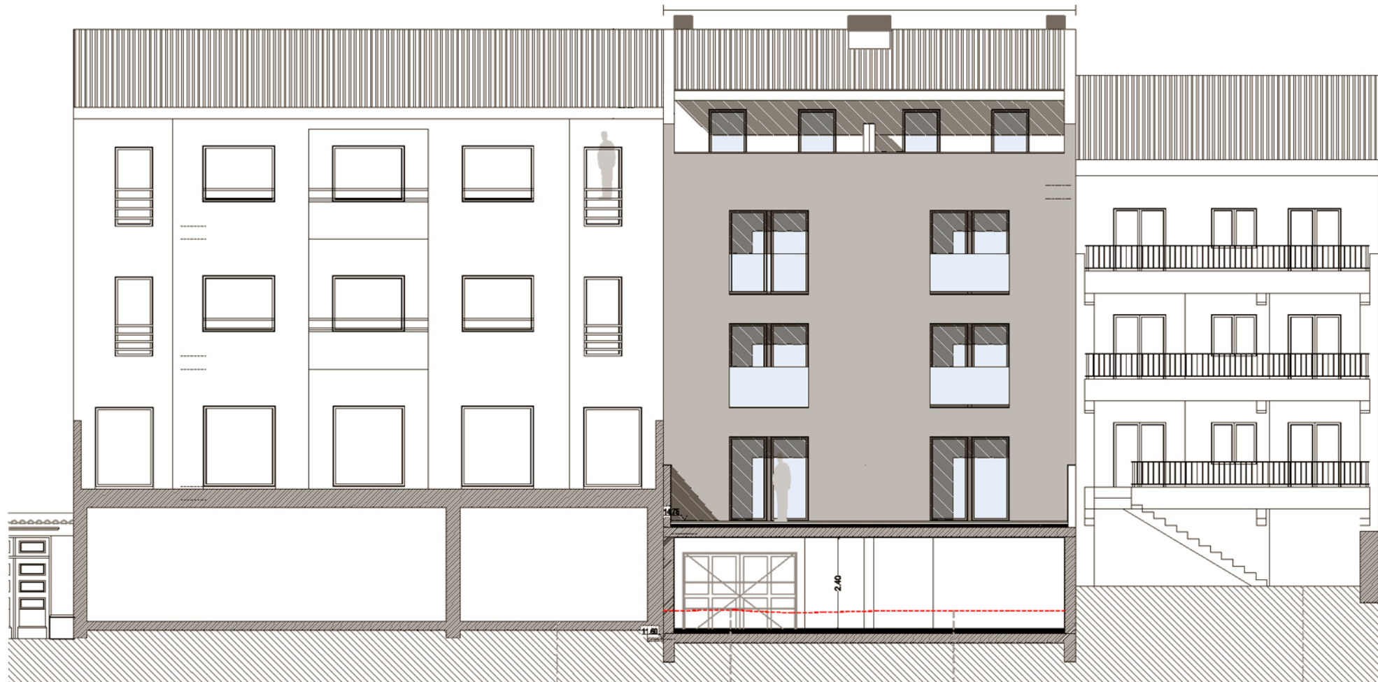
Alçado tardoz
