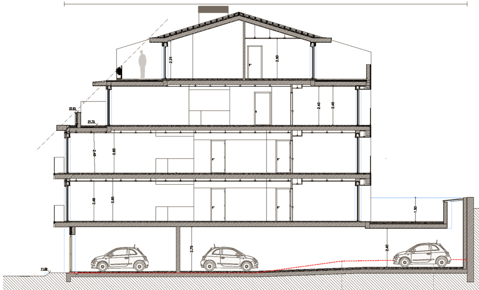
Corte
