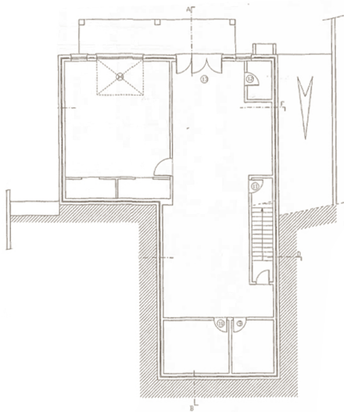
Planta da cave
