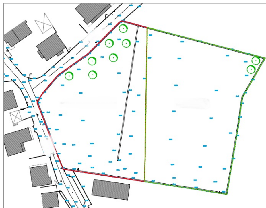
PLANTA TOPOGRÁFICA
