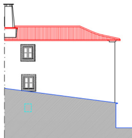
Alçado Poente
