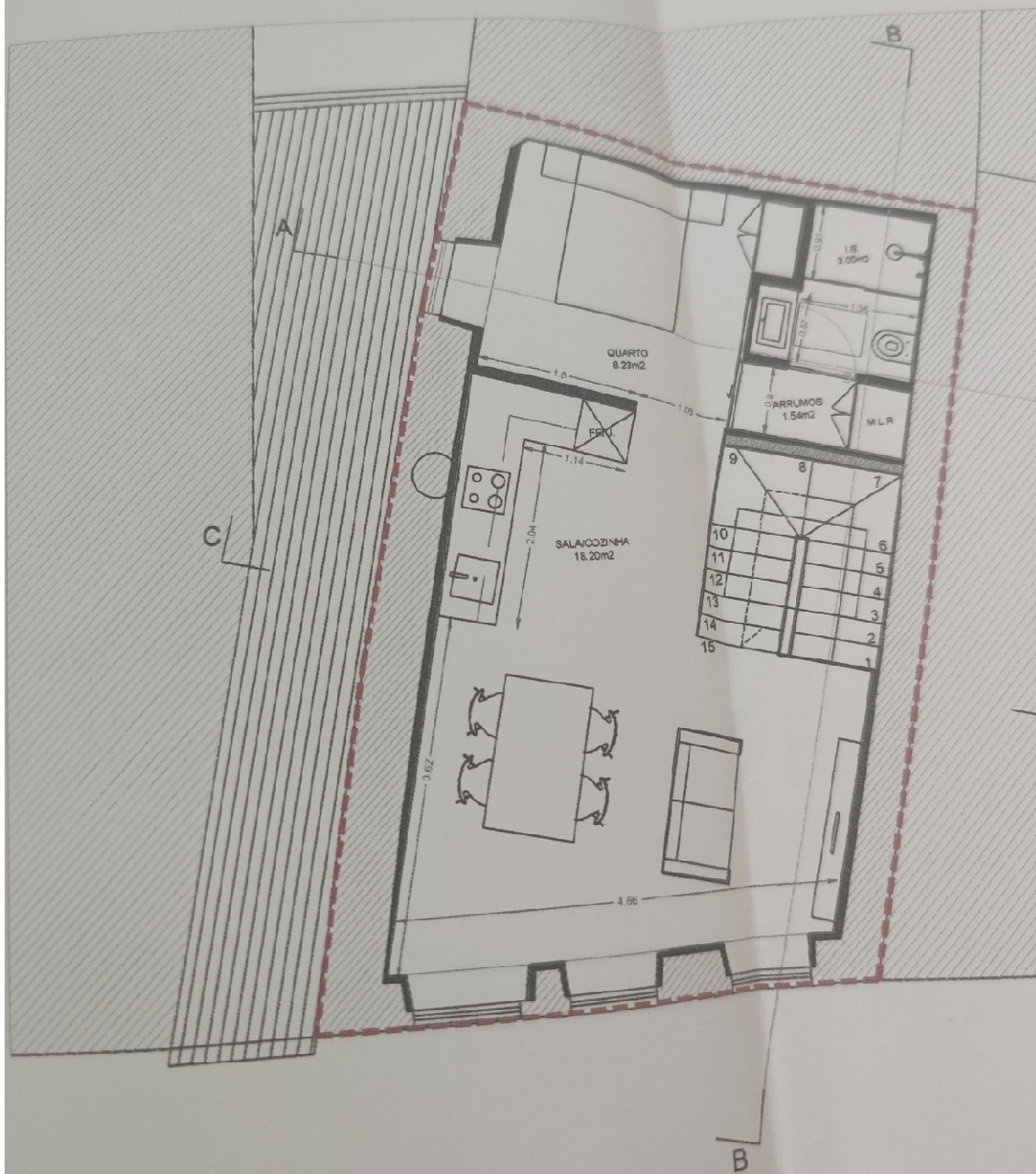
Planta do 2º Andar
