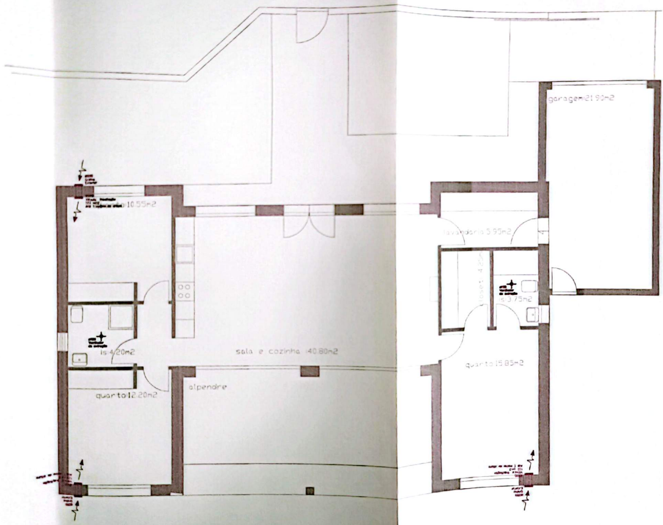
Planta do Rés do Chão
