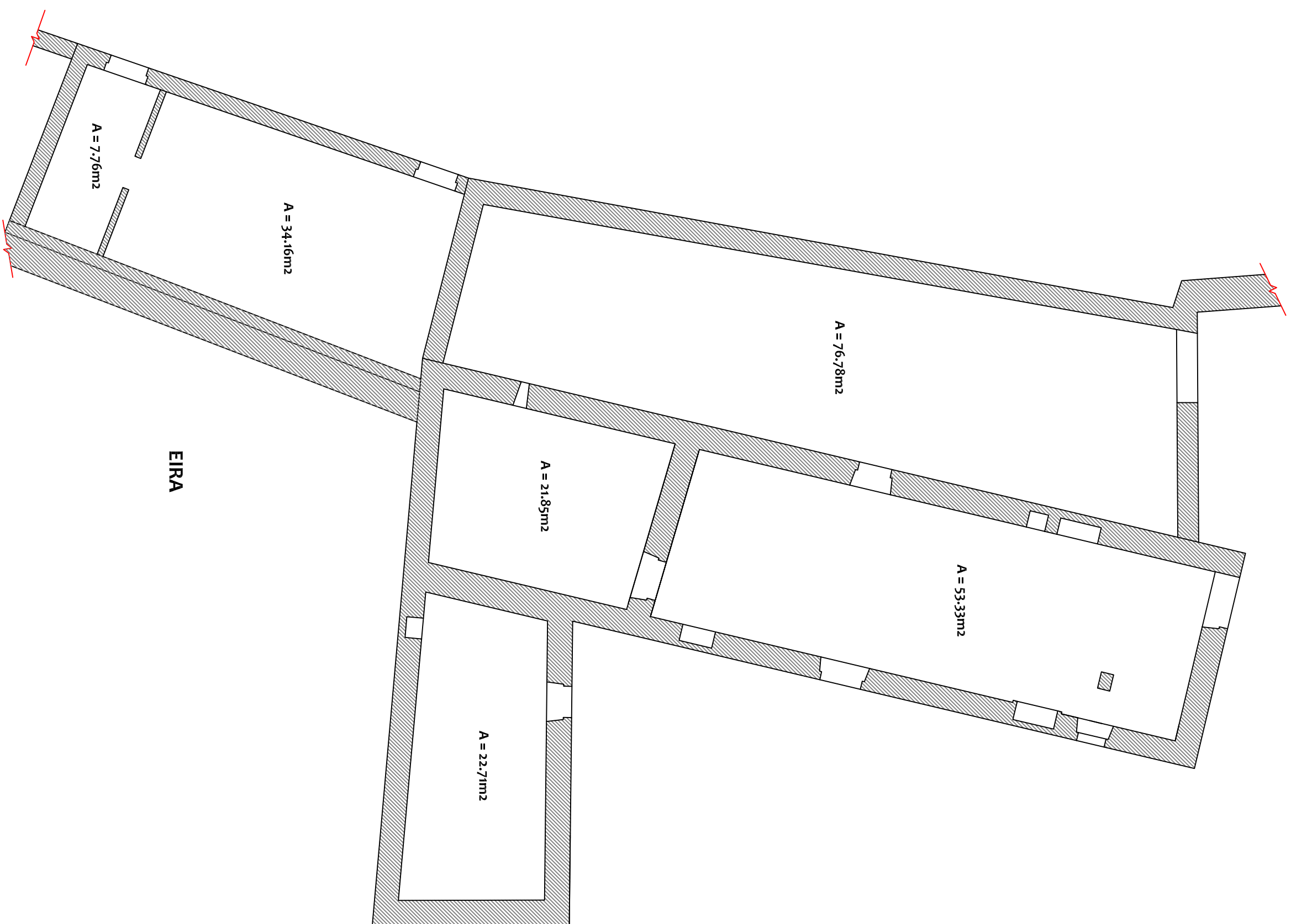
PLANTA PISO 0
