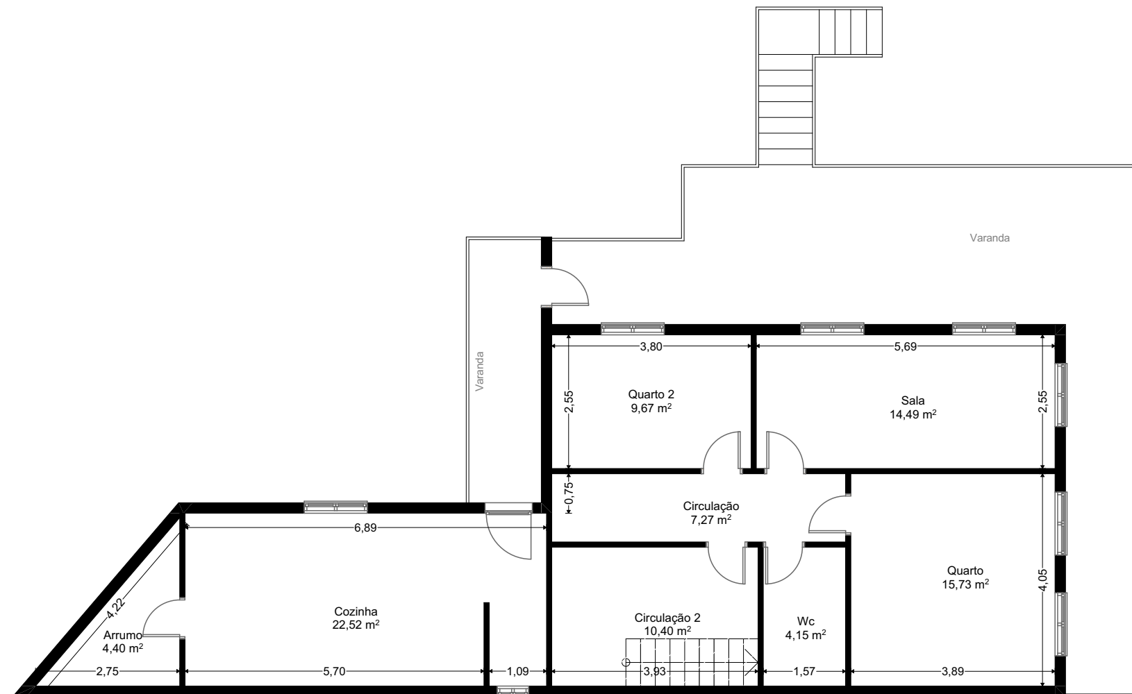
Piso 1º
