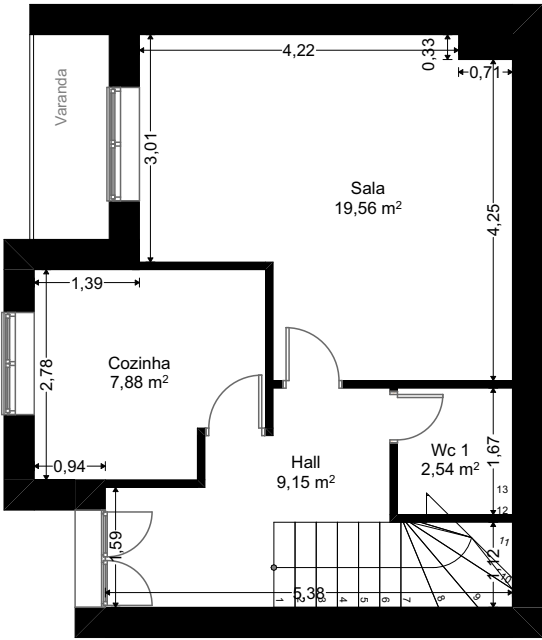
Piso Rc
